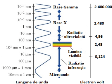
Fig. 2. Spectrul vizibil ochiului uman și radianța acestuia
