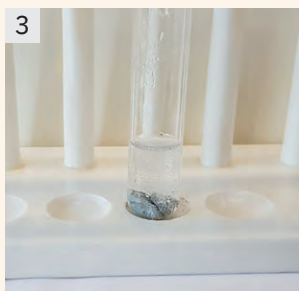
Reacția zincului cu acidul clorhidric
