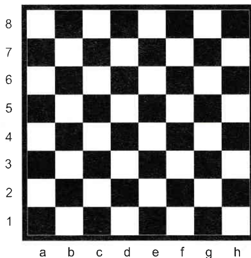
Diagrama 1: Tabla de șah
