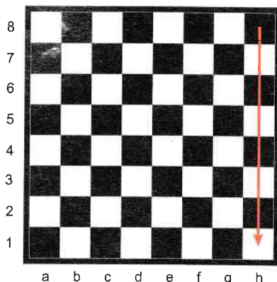
Diagrama 4: Drumul perechii regale în linie dreaptă de-a lungul coloanei h
