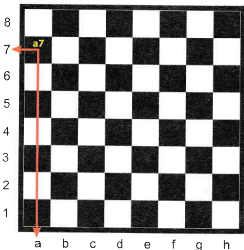
Diagrama 2: Câmpul a7
