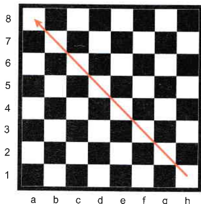
Diagrama 5: Drumul perechii regale în diagonală
