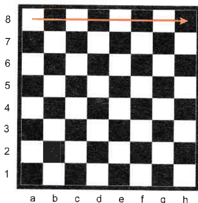
Diagrama 3: Drumul perechii regale în linie dreaptă de-a lungul rândului 8
