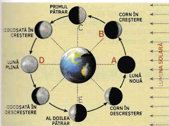
figura 1 – Fazele Lunii
