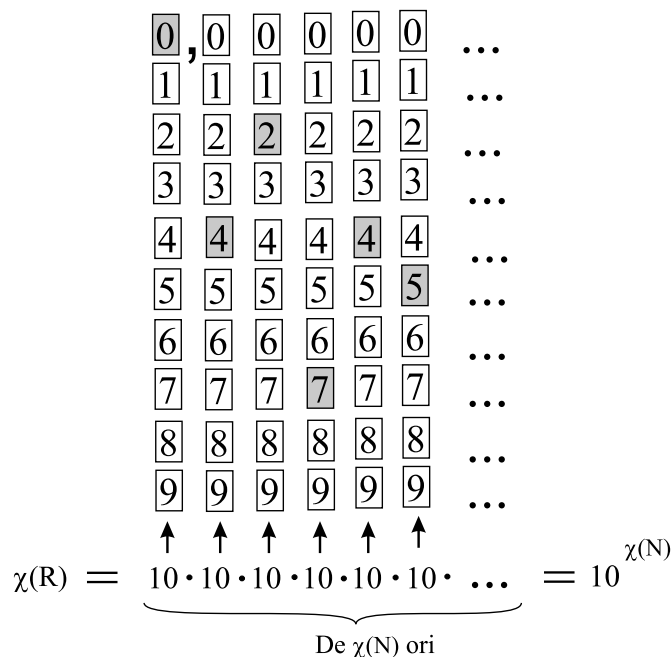
Figura 1.2: Câte numere reale avem? Pentru fiecare cifră a numărului real avem zece alegeri. În figură este exemplificat numărul real 0,42745\dots . Numărul total \chi(R) de numere reale este un produs al acestor posibilități \chi(R) = 10 \cdot 10 \cdot \dots \cdot 10 \cdot \dots . Dacă notăm cu \chi(N) numărul infinit de elemente al mulțimii numerelor naturale, atunci avem \chi(R) = 10^{\chi(N)} . Interesant este că cele două numere \chi(N) și \chi(R) sunt infinități diferite, pentru că nu poate fi găsită o relație bijectivă între mulțimile pe care le reprezintă.
