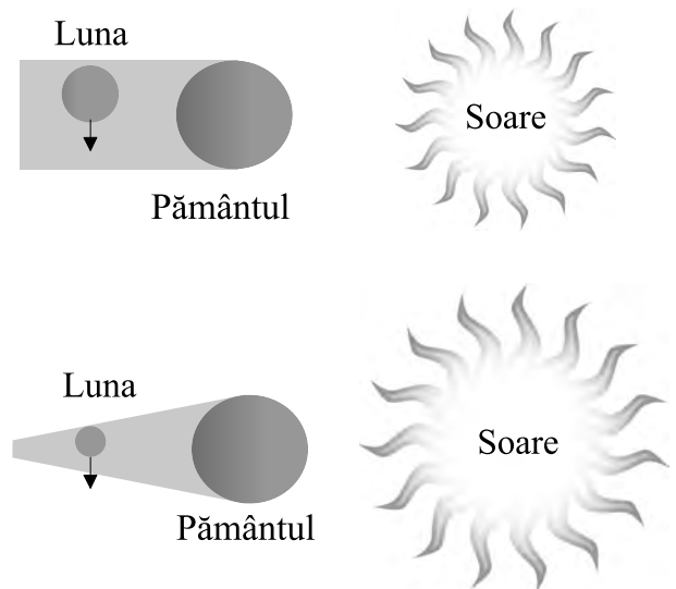
Figura 1.9: Eclipsa de Lună în interpretarea lui Aristarh (sus) și în interpretarea modernă corectă (jos). În ambele cazuri Luna intră în conul de umbră al Pământului, atâta doar că Aristarh credea că umbra are o formă cilindrică.
